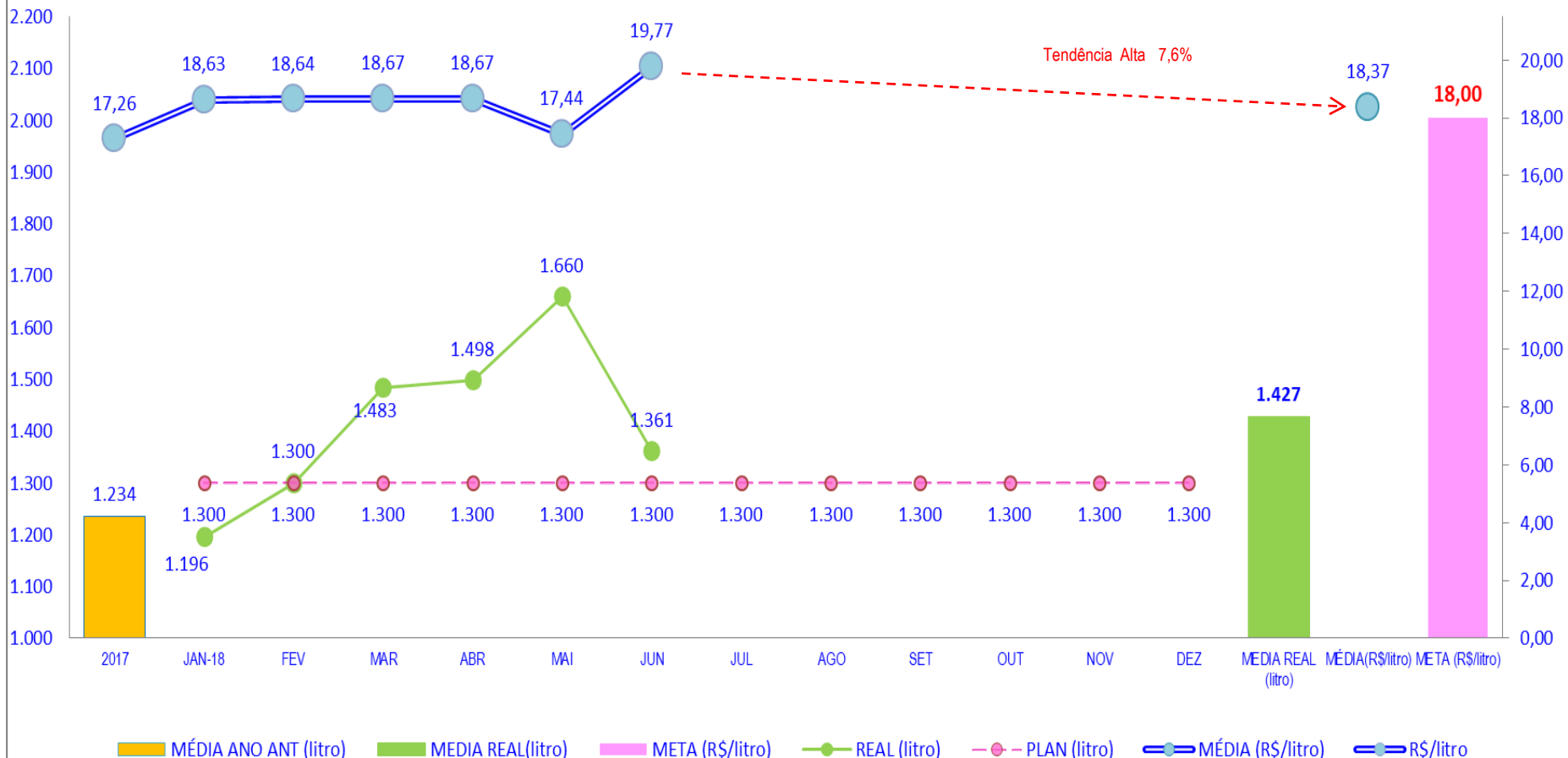
Evolução Tratamento e Custo de Esgoto Samae (DJ) - 2018
